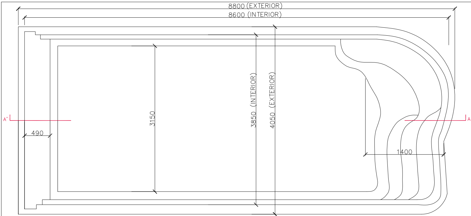
PLANTA
