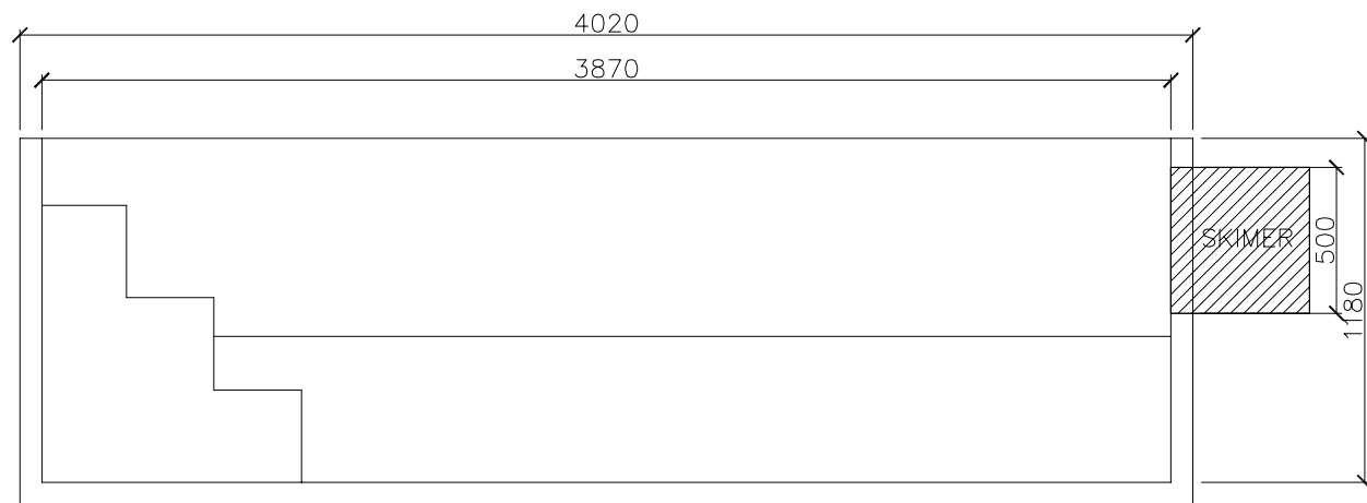
SECCIÓN A-A'
