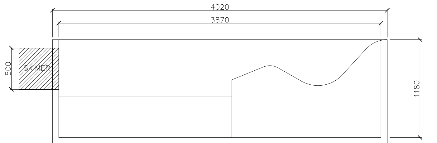
SECCIÓN B-B'
